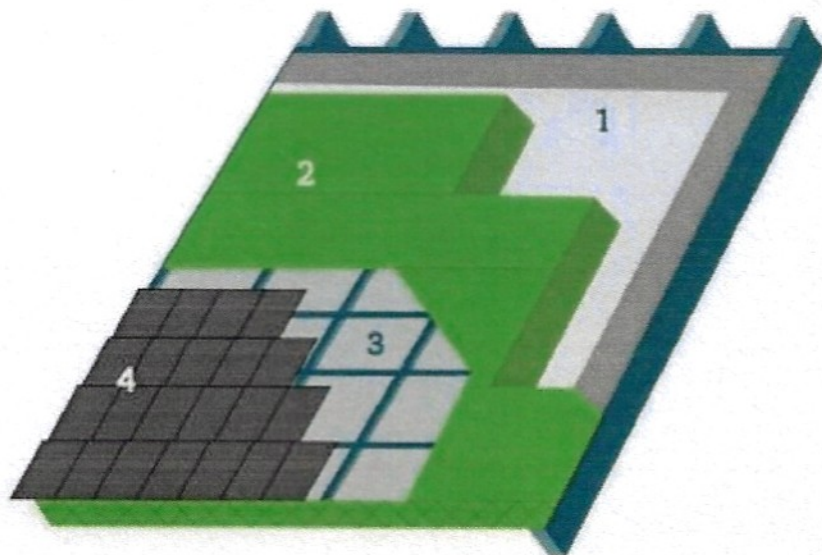
1. Dampscherm | 2. Isolatie | 3. Onderdak | 4. Dakbekleding
