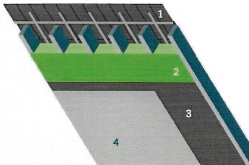
1. Onderdak | 2. Isolatie | 3. Dampscherm | 4. binnenafwerking
